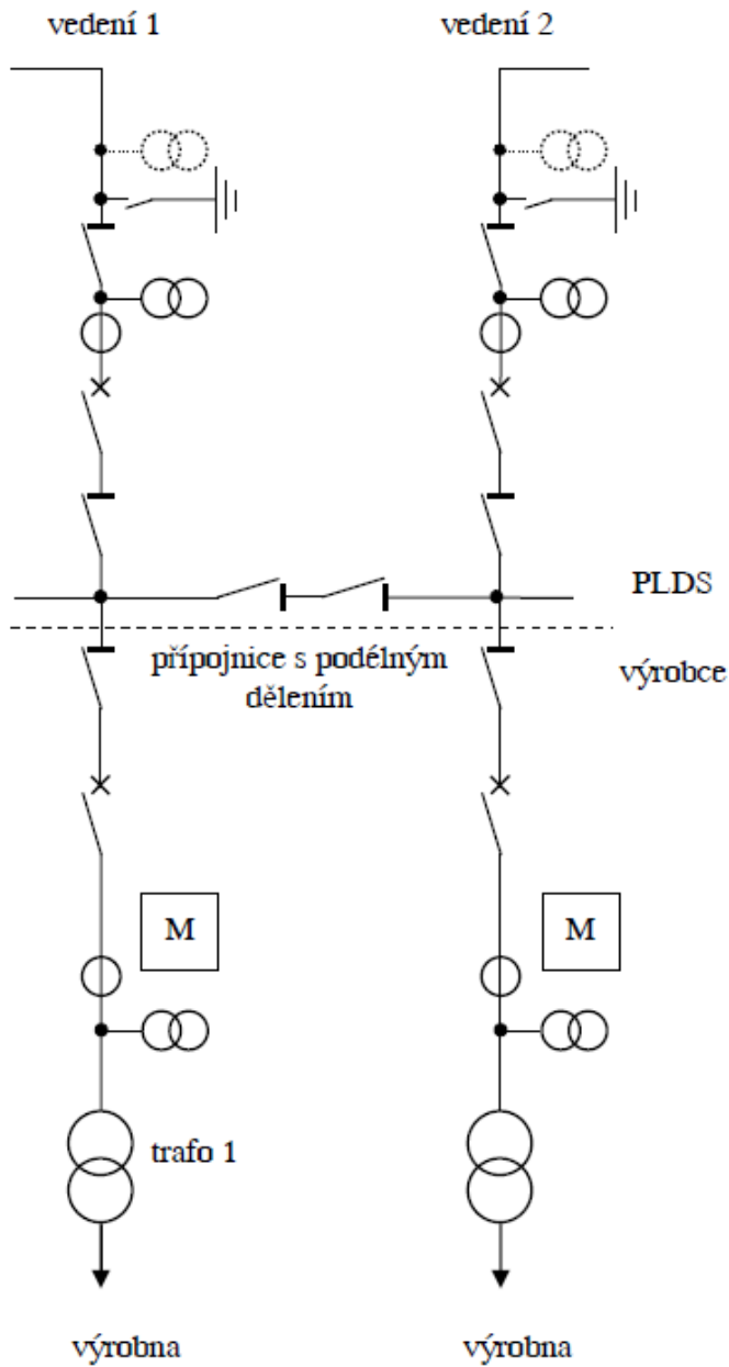
Obr. 14 Připojení výrobní zasmyčkováním do vedení 110 kV LDS
